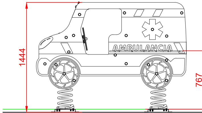
ALZADO
