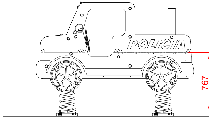
ALZADO
