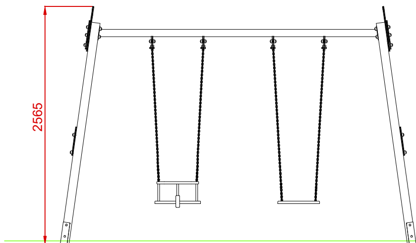
ALZADO
