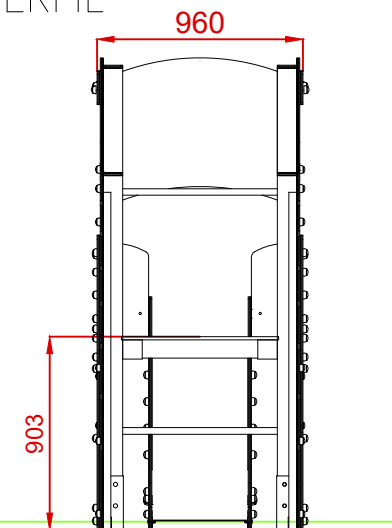
PERFIL
