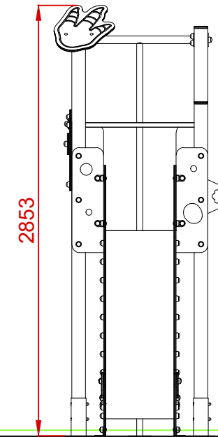
PERFIL IZQUIERDO
