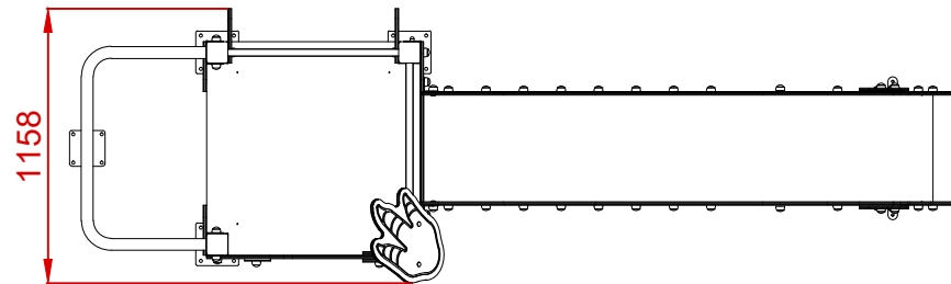
PLANTA
