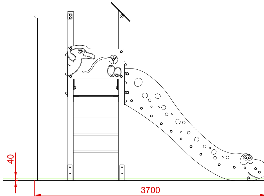
ALZADO
