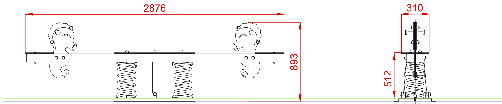
ALZADO
