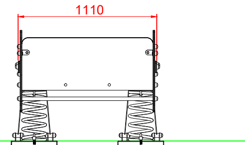
PERFIL
