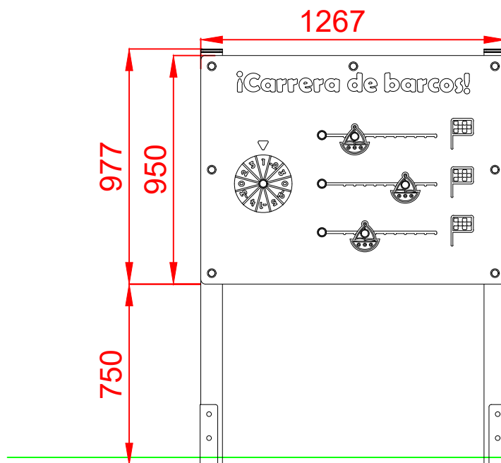
ALZADO
