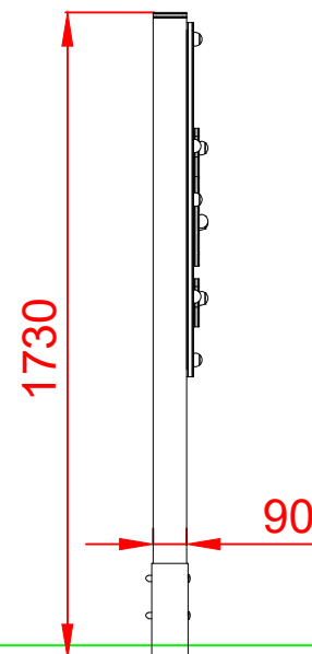
PERFIL IZQUIERDO
