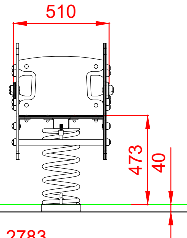
PERFIL
