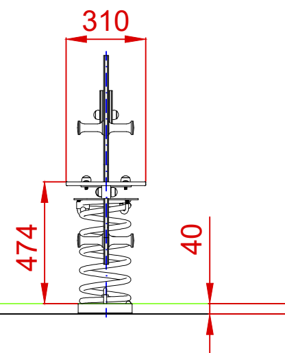
PERFIL
