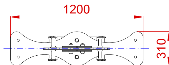
PLANTA
