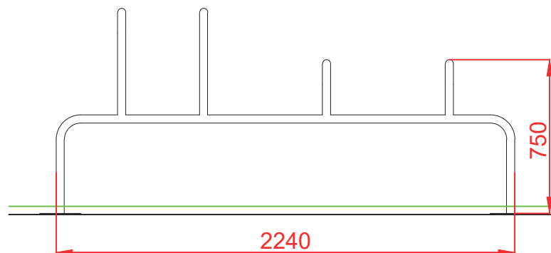
ALZADO
