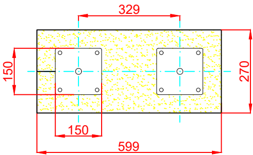
PLANTA DE CIMENTACIÓN E: 2/1
