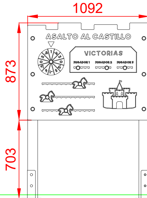
ALZADO
