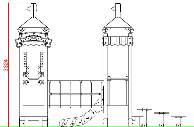
PERFIL
