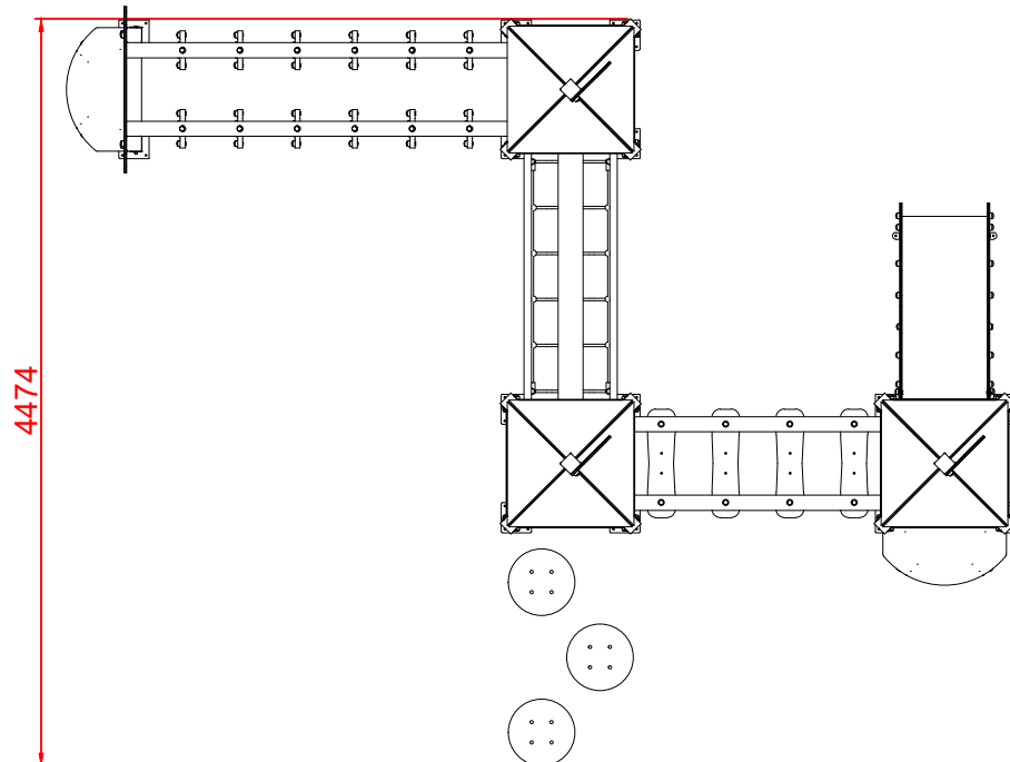
PLANTA
