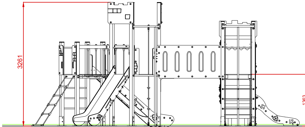
ALZADO
