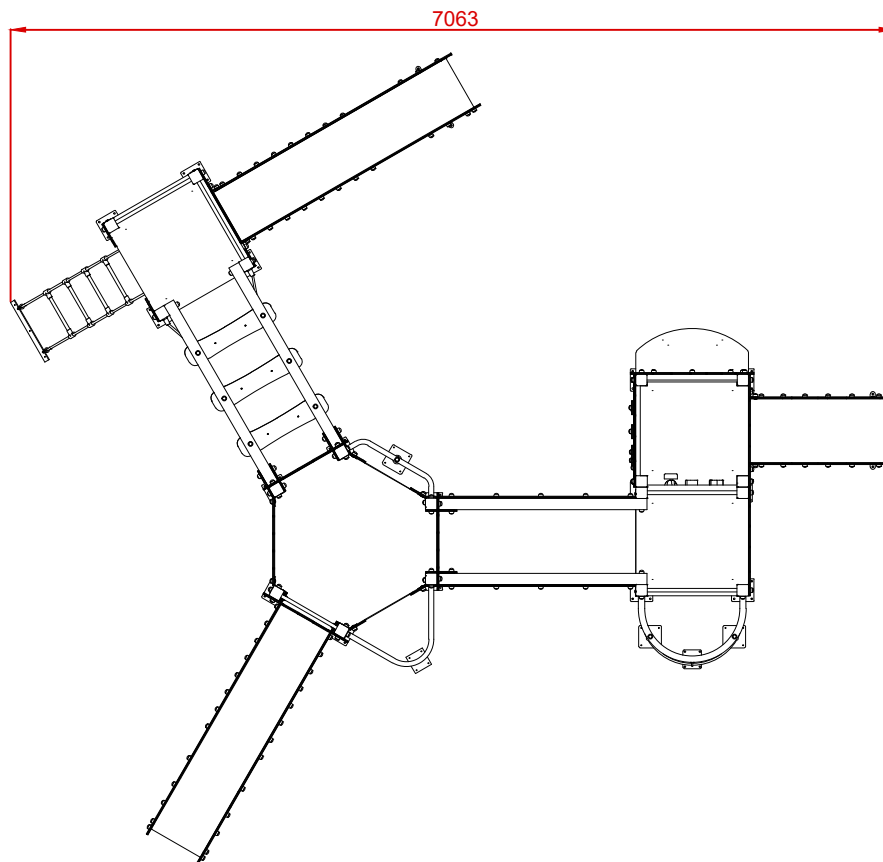
PLANTA
