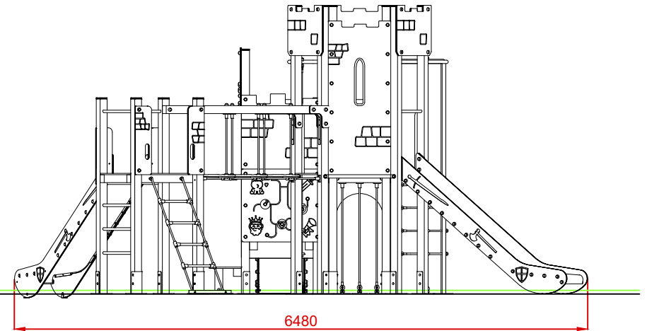
PERFIL IZQUIERDO
