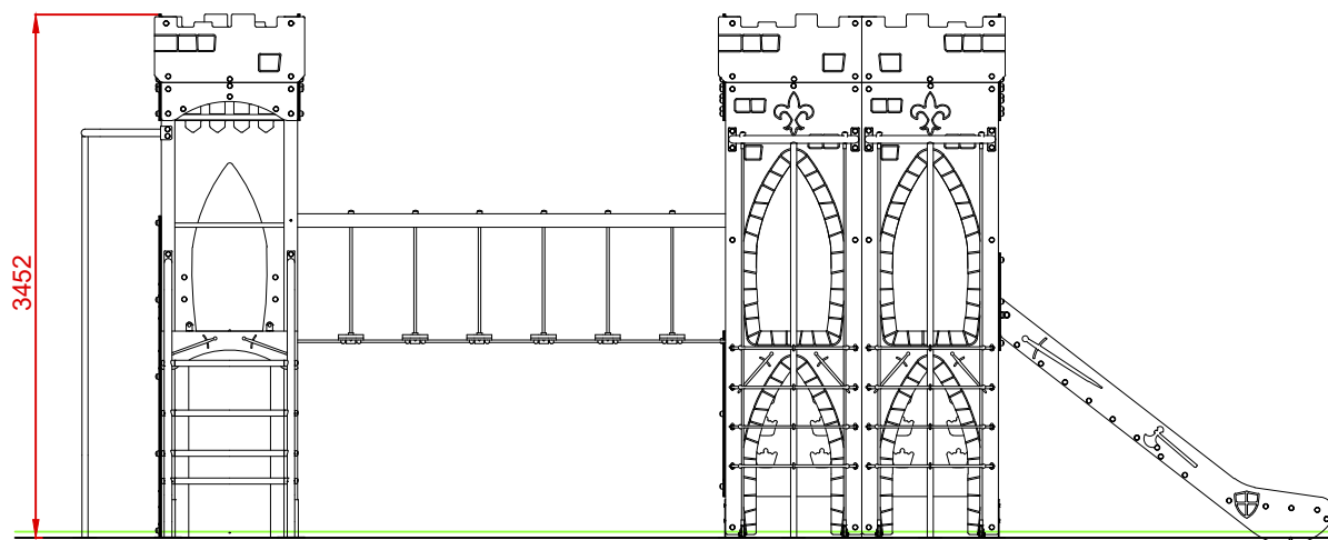
ALZADO
