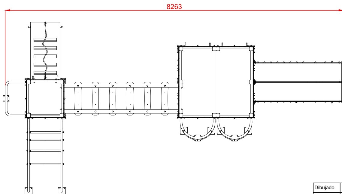
PLANTA
