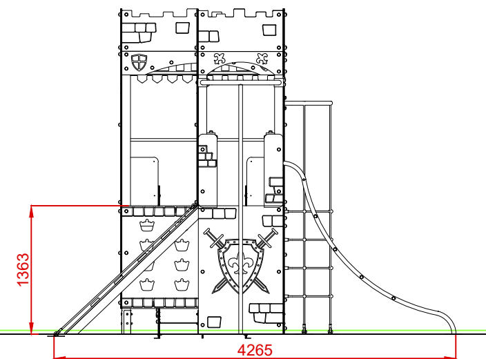
PERFIL IZQUIERDO
