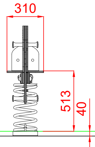
PERFIL
