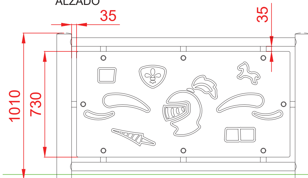
ALZADO
