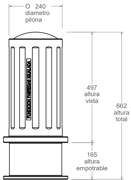
vista alzado 1:10
