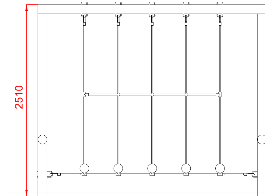
ALZADO
