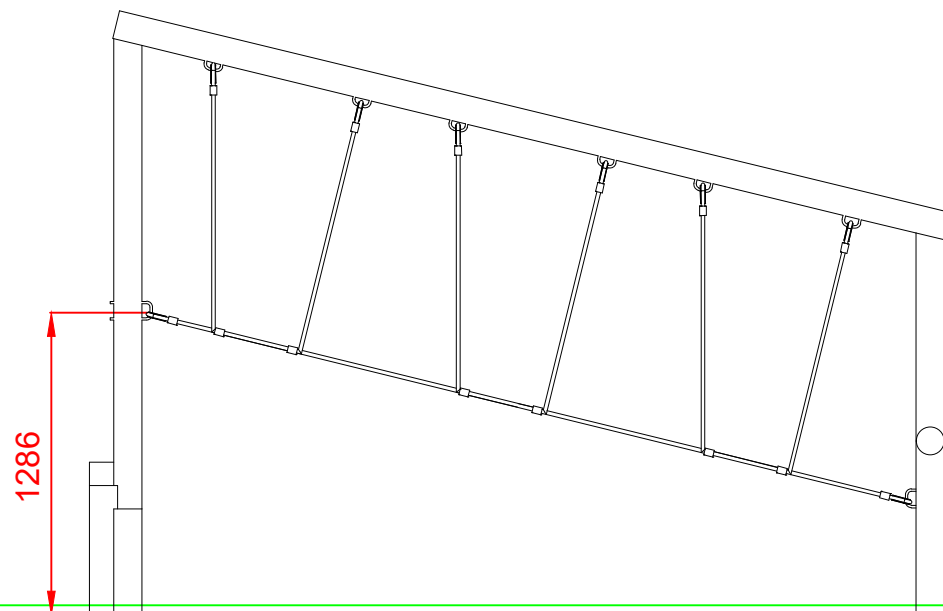
ALZADO
