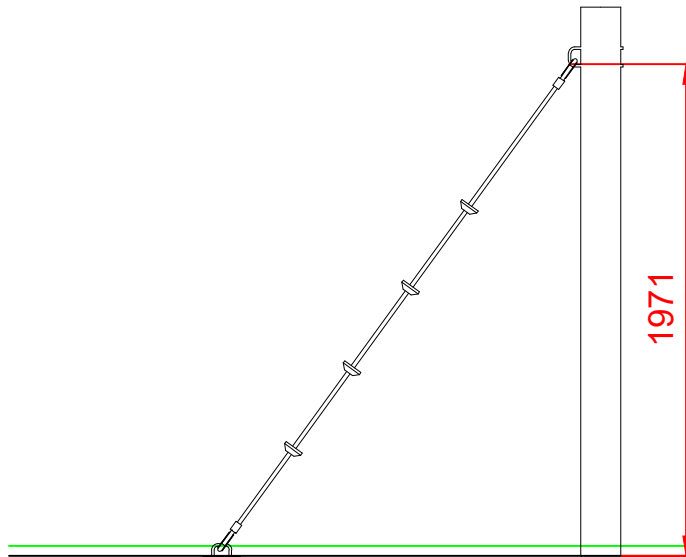
ALZADO
