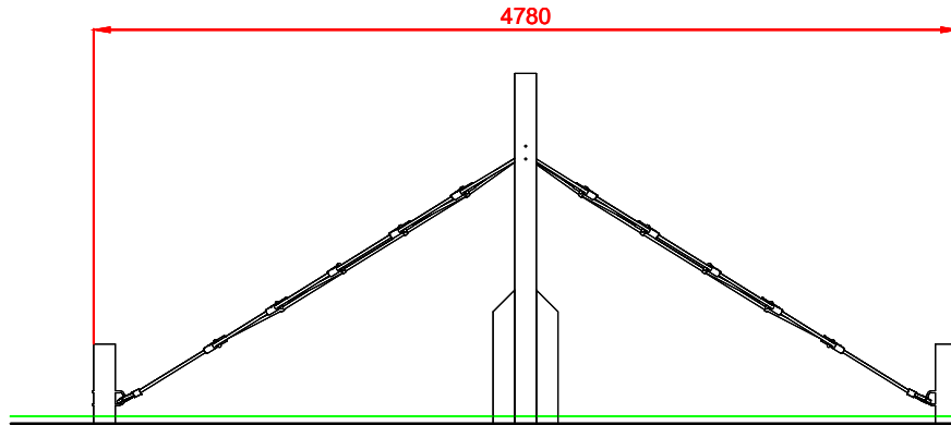
ALZADO
