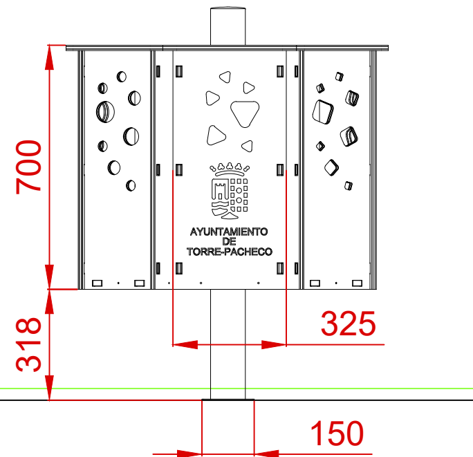
PERFIL IZQUIERDO
