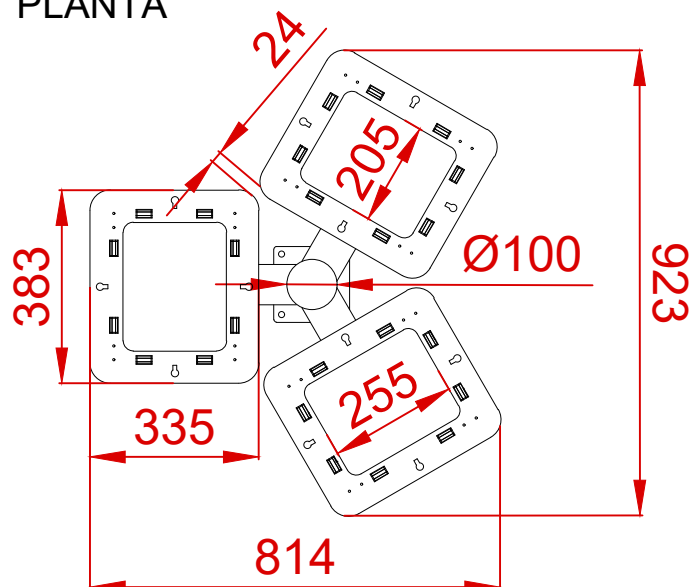
PLANTA
