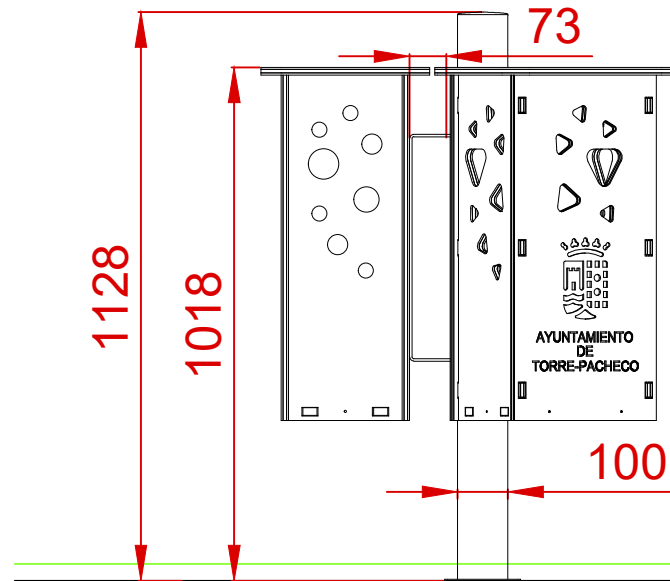
ALZADO
