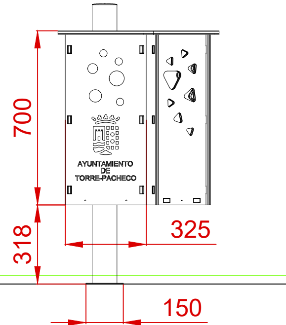
PERFIL IZQUIERDO
