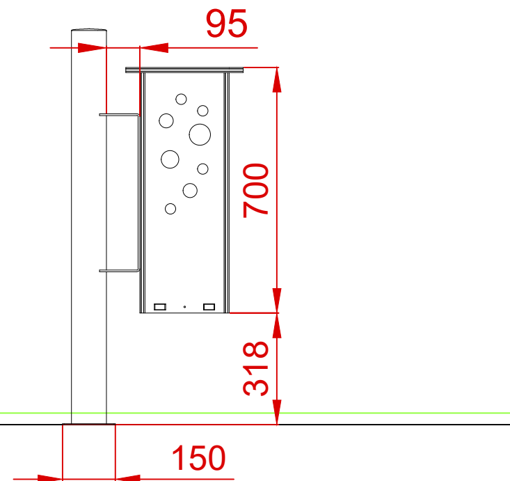
PERFIL IZQUIERDO
