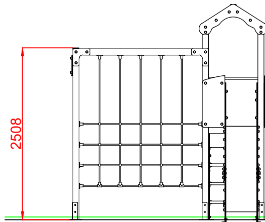
ALZADO
