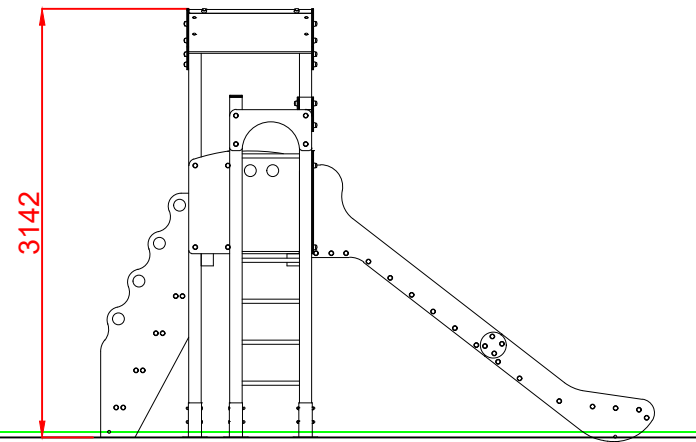
PERFIL
