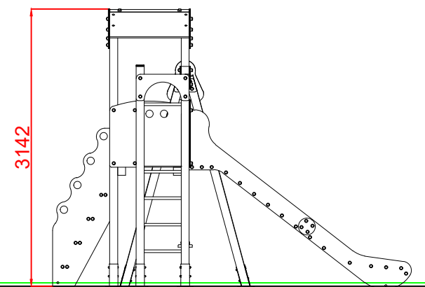
PERFIL
