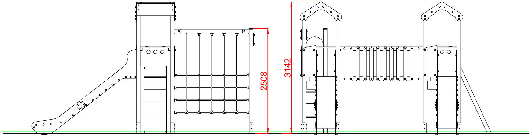
ALZADO
