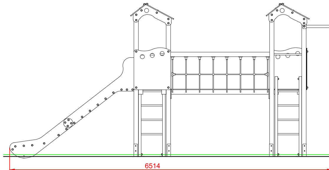
ALZADO
