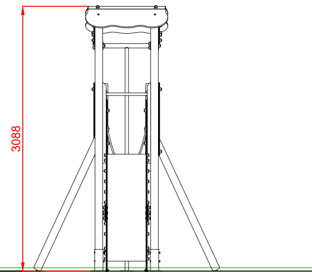
PERFIL IZQUIERDO
