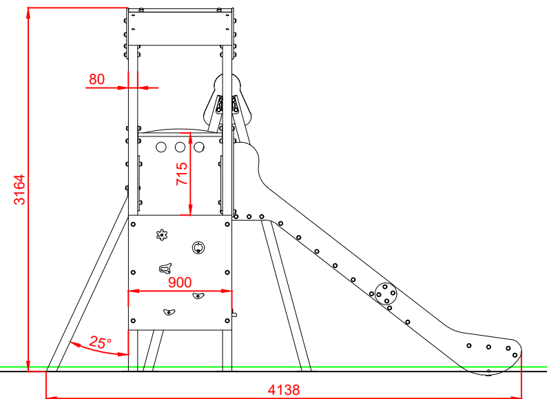
PERFIL IZQUIERDO
