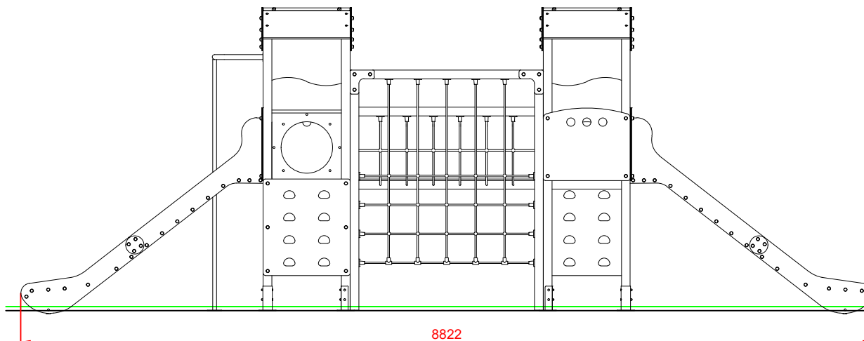
ALZADO
