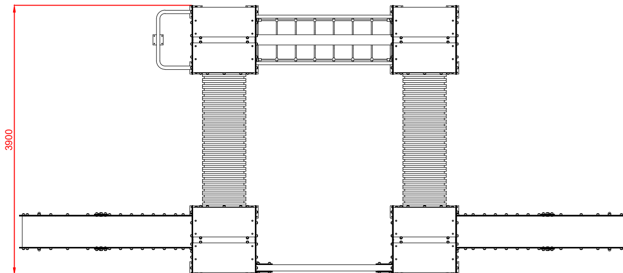
PLANTA
