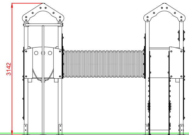
PERFIL IZQUIERDO
