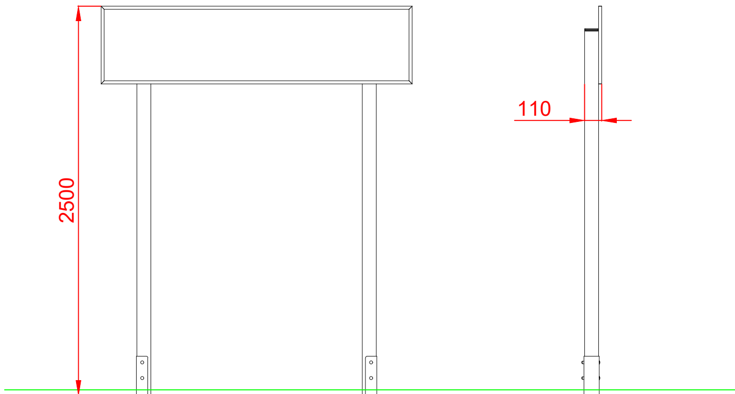
ALZADO
