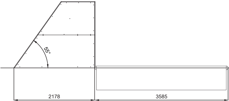
PLANTA
