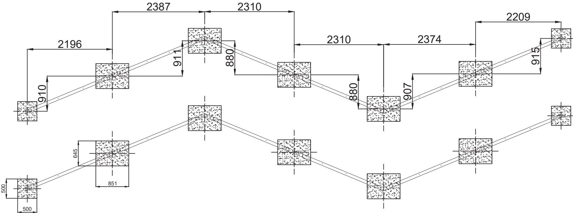
ESQUEMA DE CIMENTACIÓN POSTES
