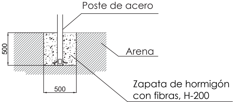
ESQUEMA DE CIMENTACIÓN POSTES
