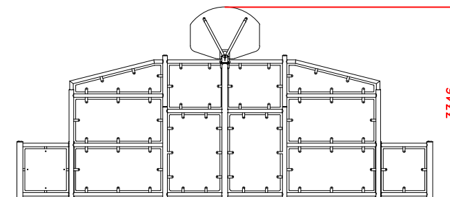
ALZADO
