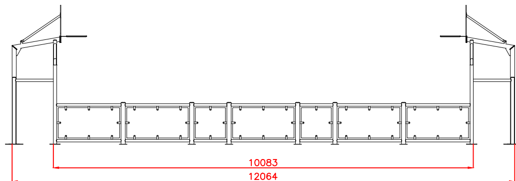
PERFIL IZQUIERDO
