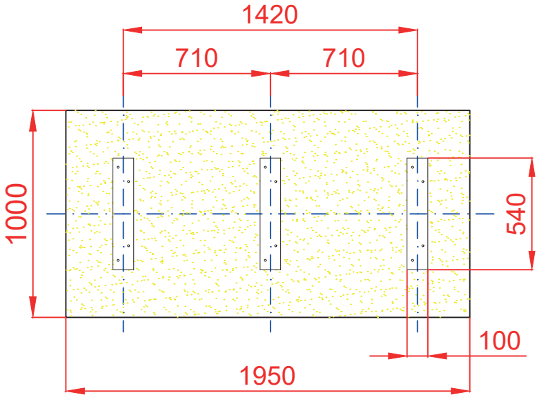
PLANTA CIMENTACIÓN
