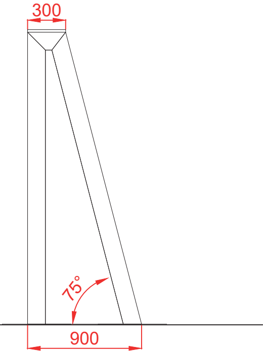
PERFIL IZQUIERDO
