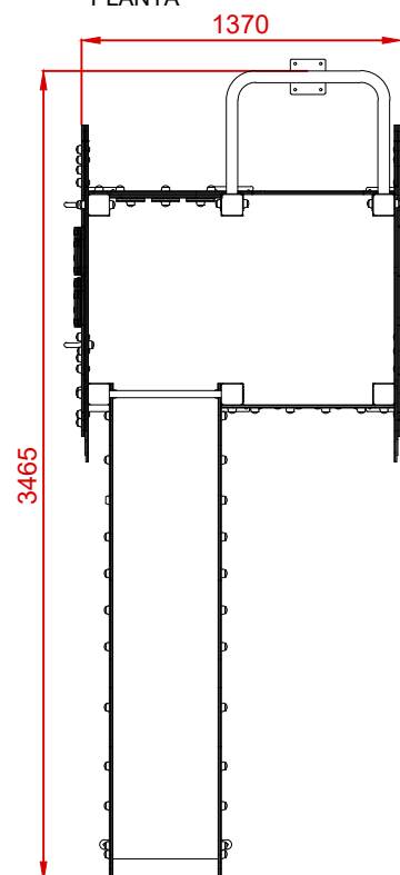
PLANTA
