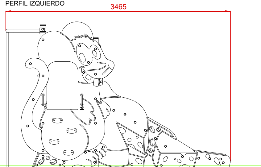
PERFIL IZQUIERDO
