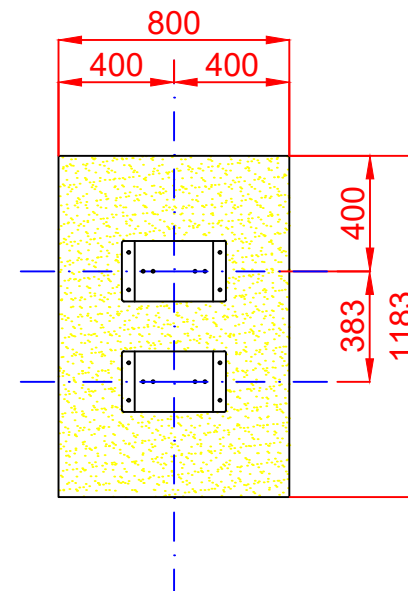
PLANO DE CIMENTACIÓN
