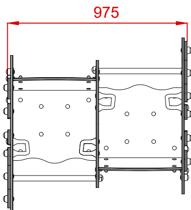
PLANTA
