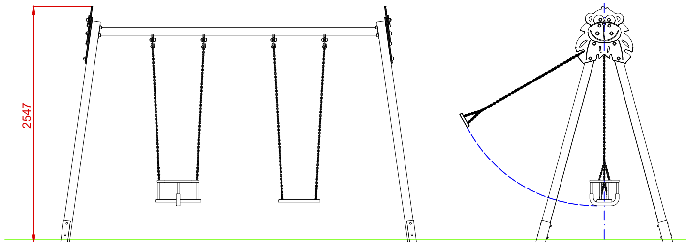
ALZADO
