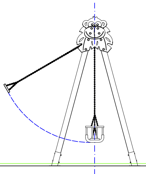
PERFIL IZQUIERDO
