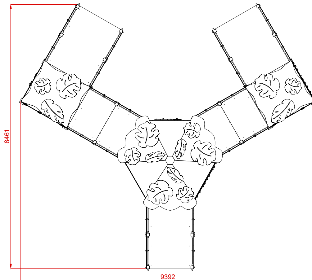
PLANTA
