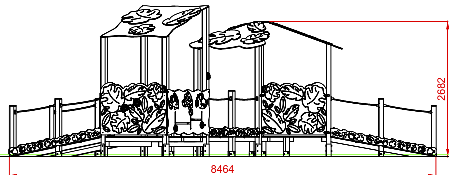
PERFIL IZQUIERDO
