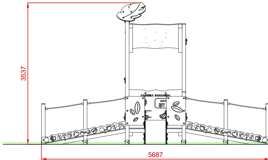
ALZADO
