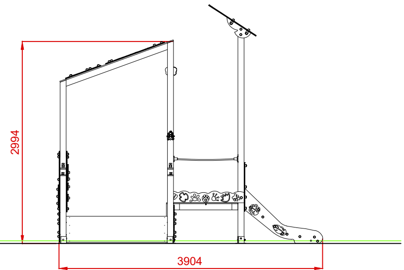
PERFIL IZQUIERDO
