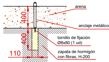
ESQUEMA DE CIMENTACIÓN EN HORMIGÓN
