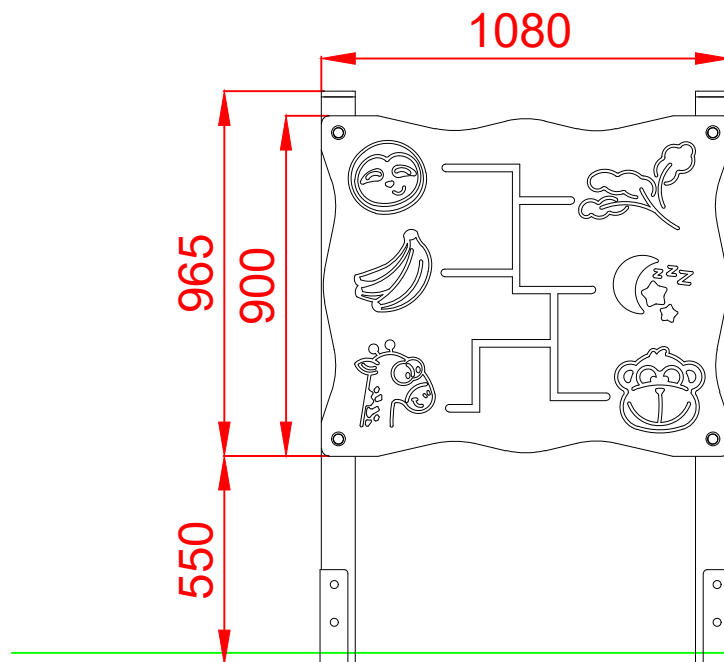
ALZADO
