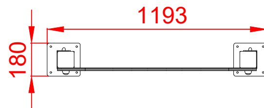
PLANTA
