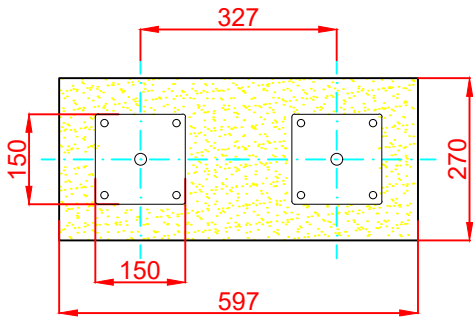
PLANTA DE CIMENTACIÓN E: 2/1
