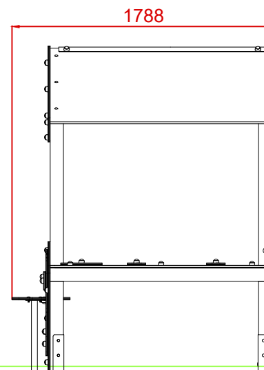
PERFIL IZQUIERDO
