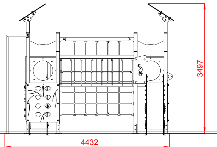
PERFIL IZQUIERDO
