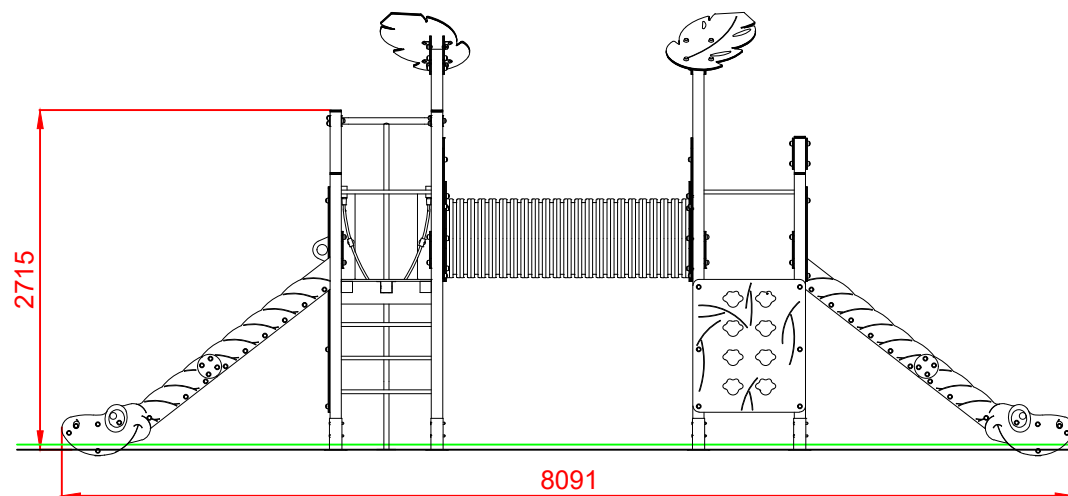
ALZADO
