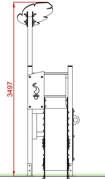
PERFIL IZQUIERDO
