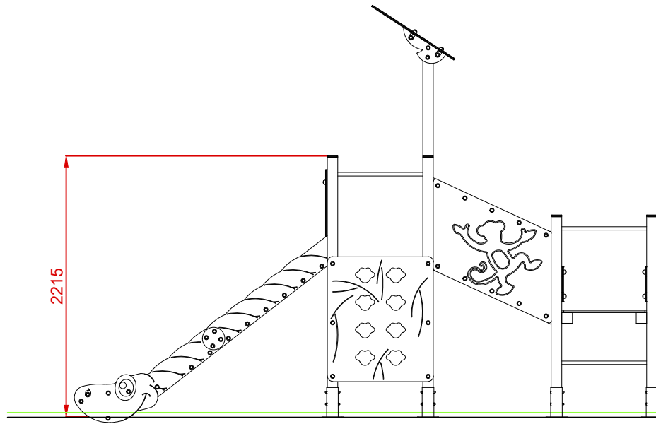
ALZADO
