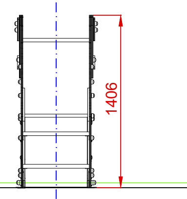
PERFIL IZQUIERDO
